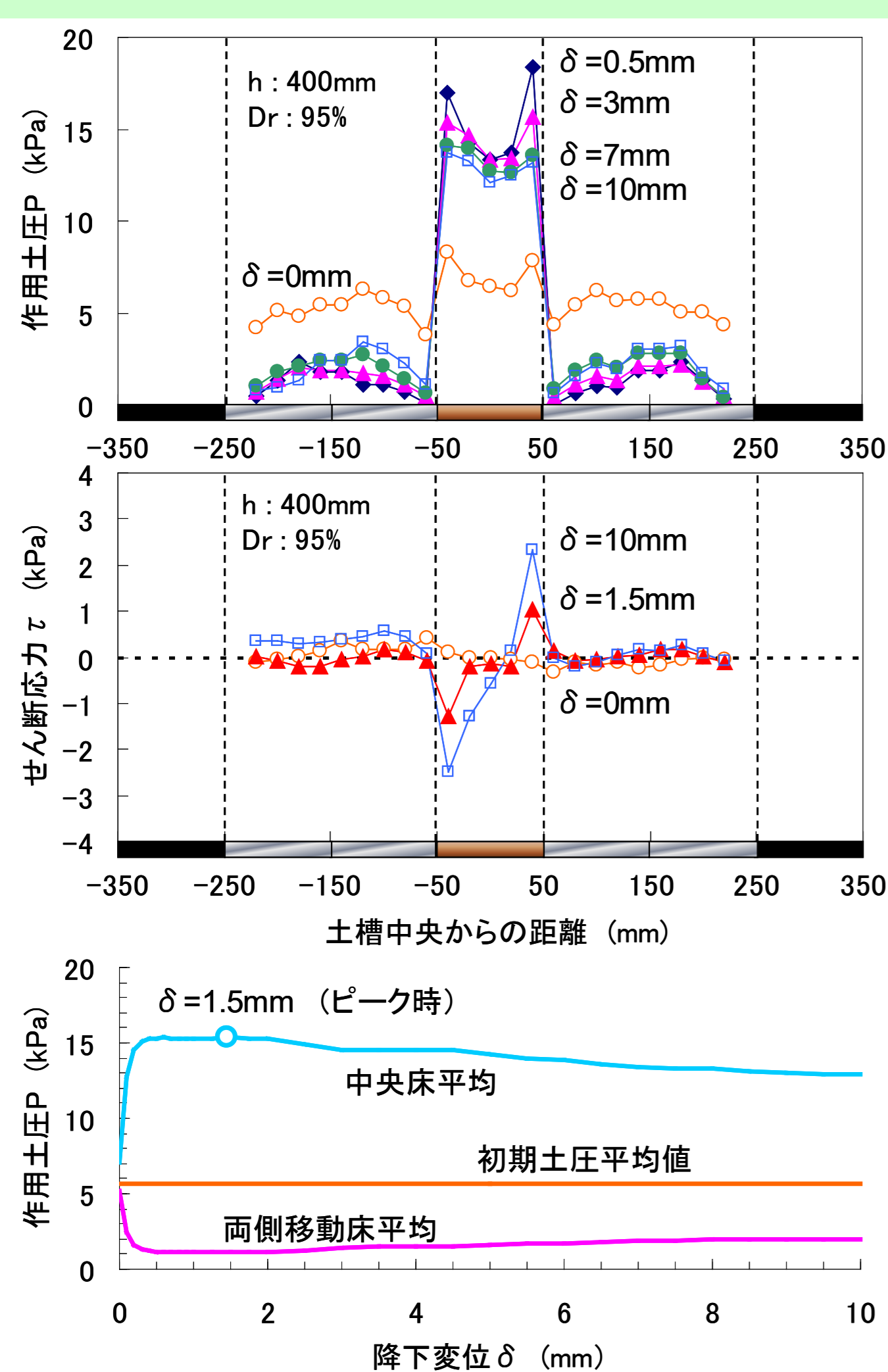
移動床実験における底板の作用土圧(豊浦砂密詰) Trapdoor test results on densely compacted Toyoura sand
