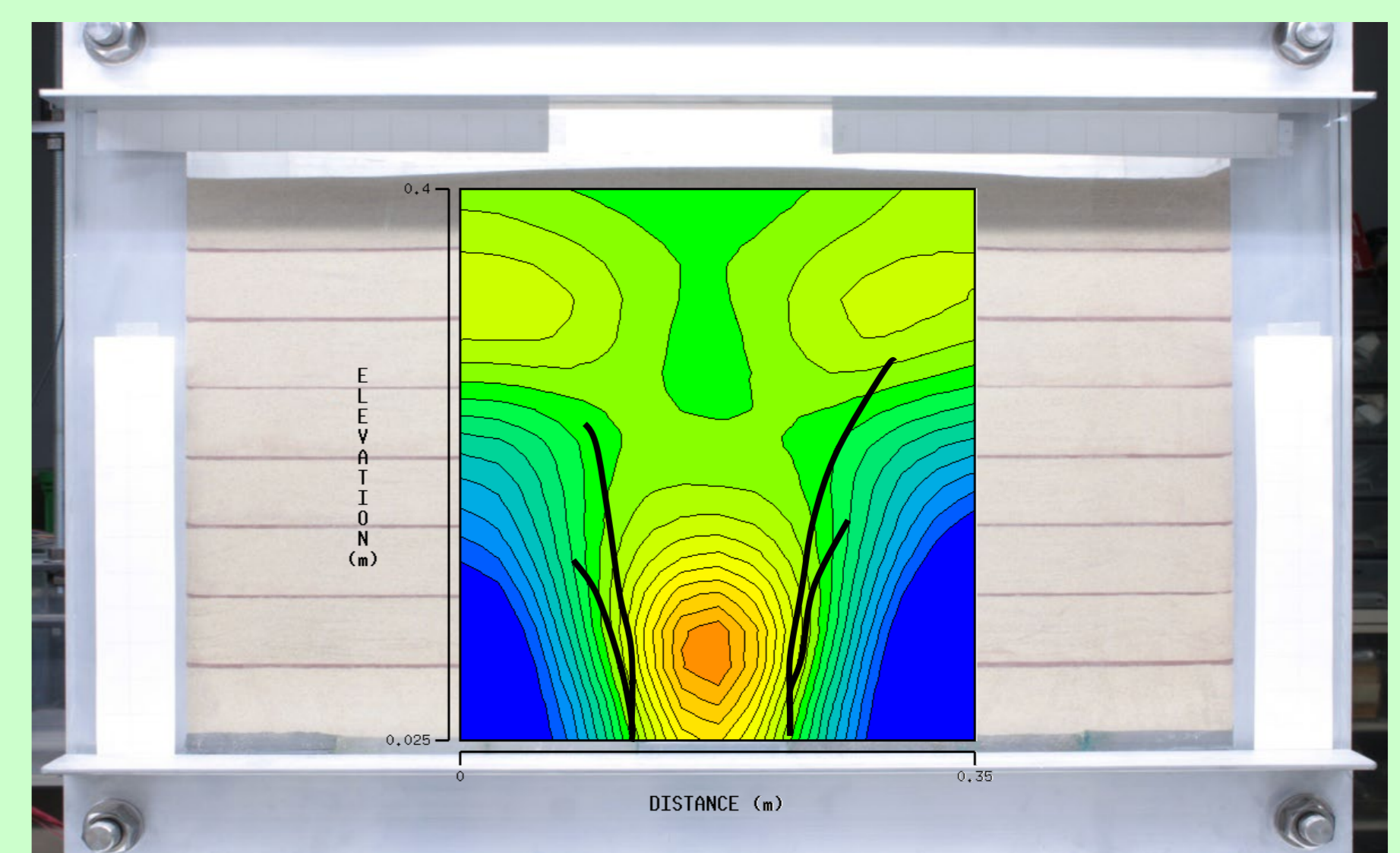
移動前後の速度差分布と地盤のすべり線
